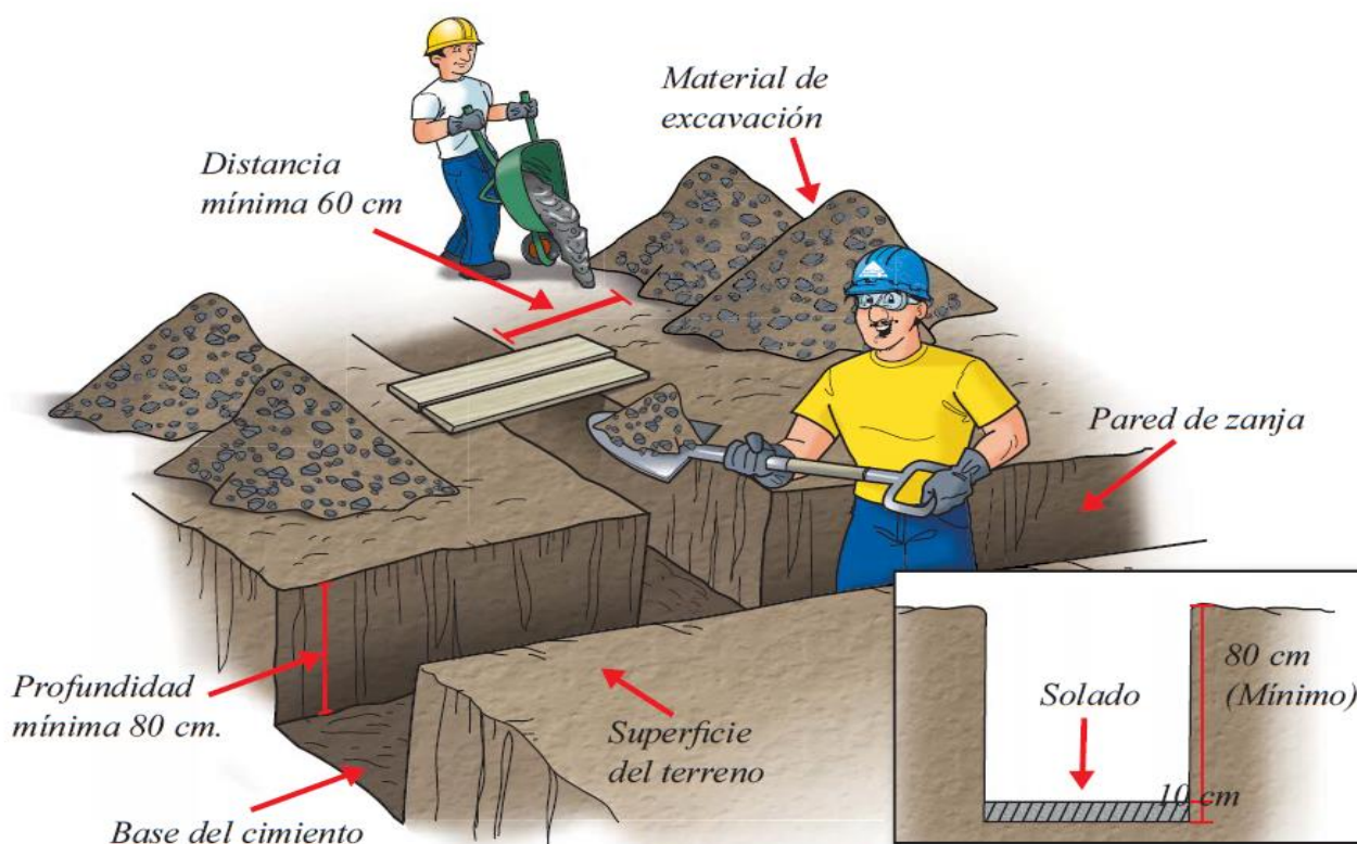
SECCIÓN TRANSVERSAL DE LA ZANJA
