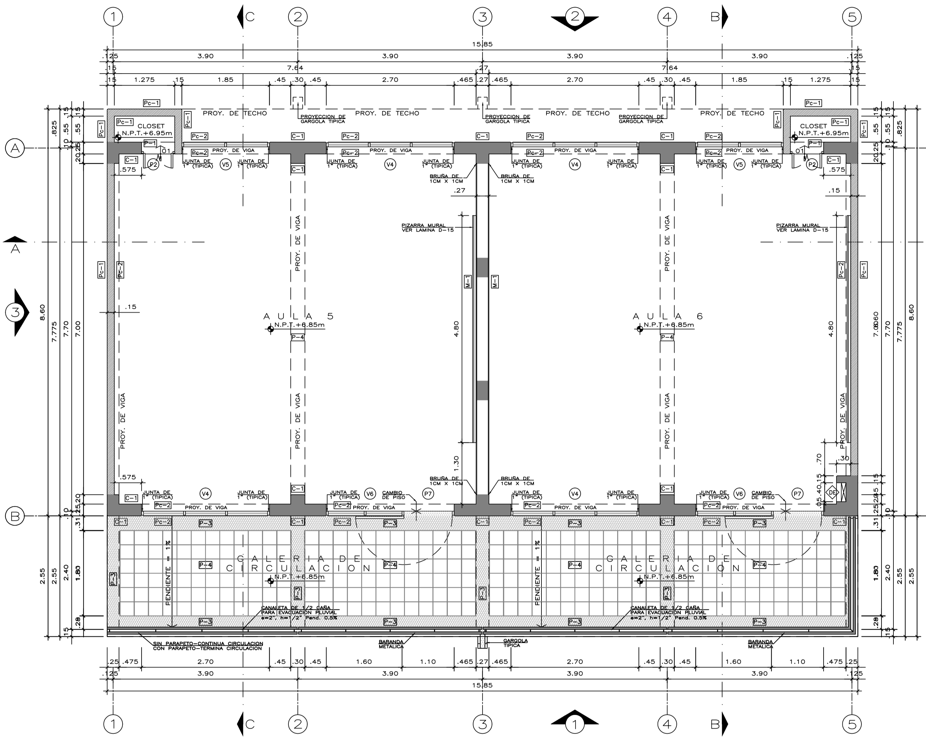
PLANTA TERCER PISO ESCALA 1/50
