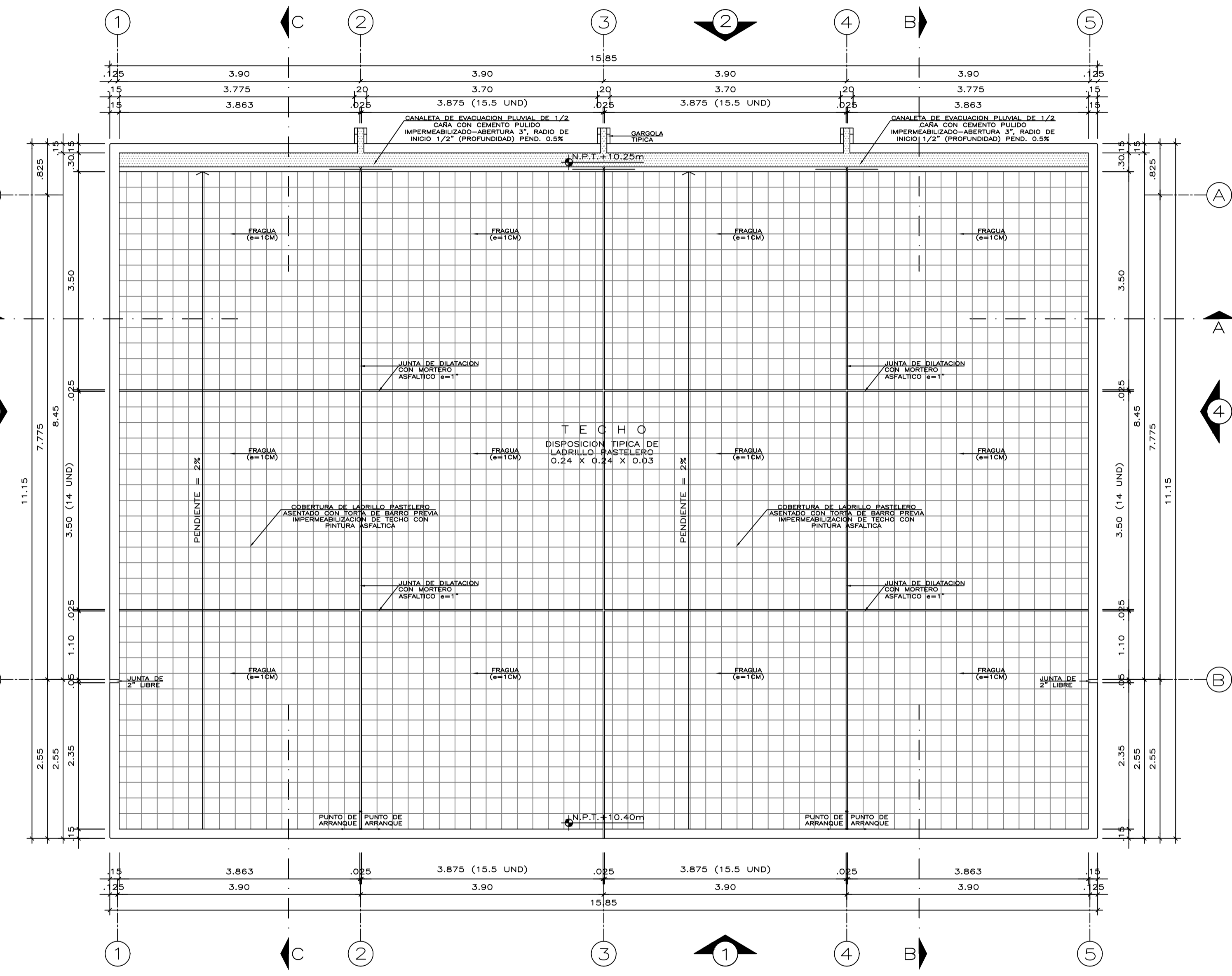
PLANTA DE TECHO ESCALA 1/50
