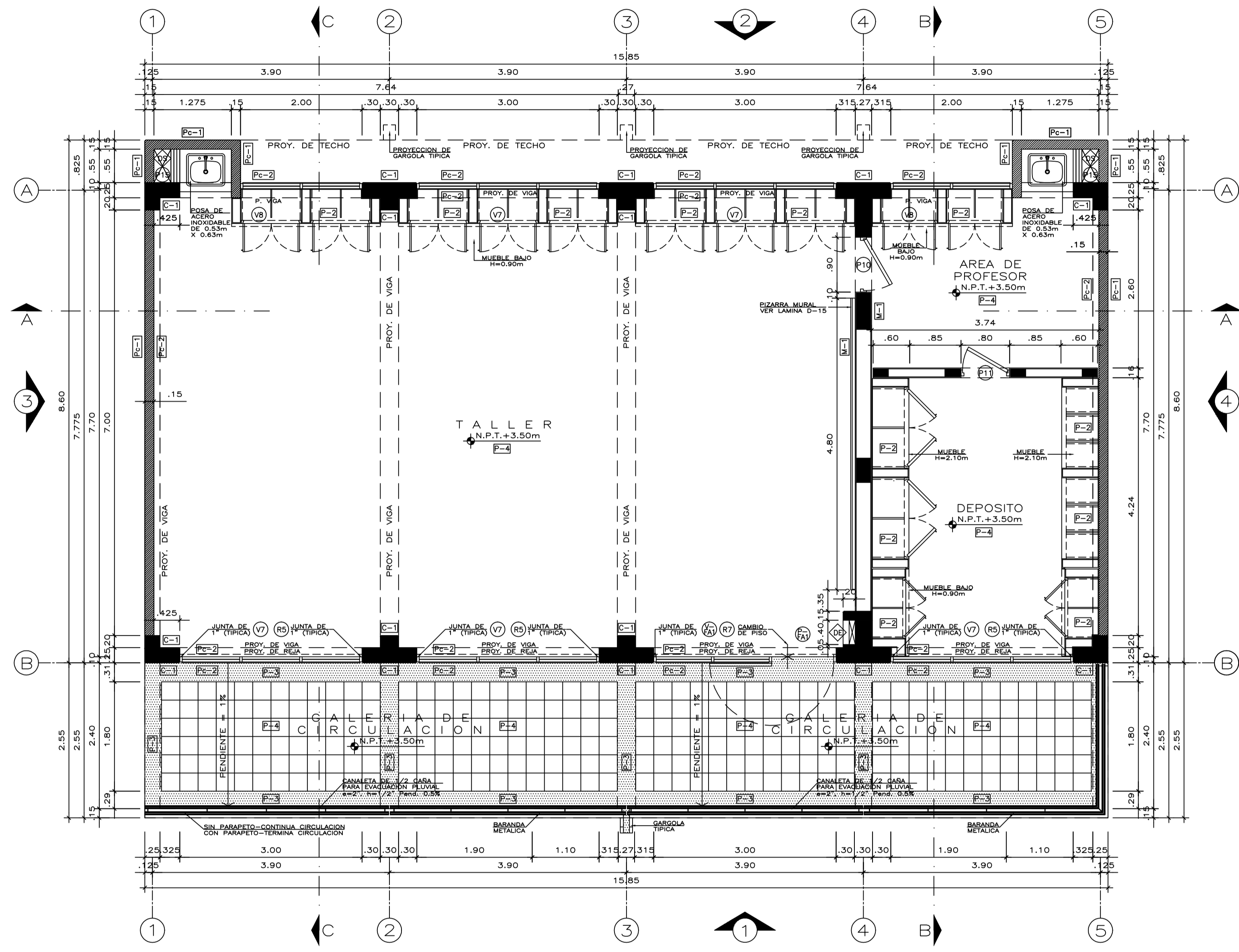
PLANTA SEGUNDO PISO ESCALA 1/50
