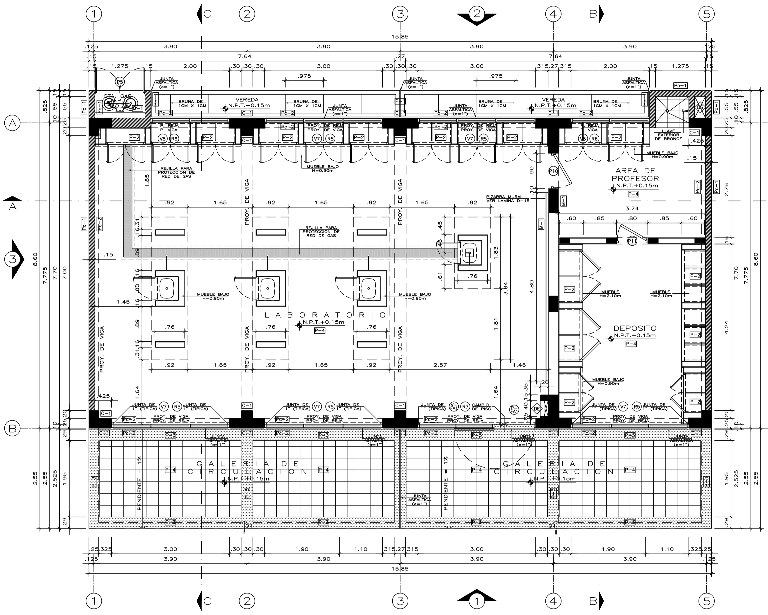
PLANTA PRIMER PISO ESCALA 1/50
